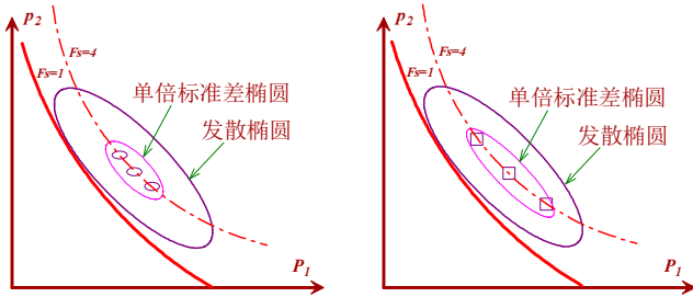
图 5 相同安全系数下得到可靠度指标明显差异
