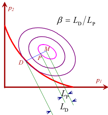
图3 设计点、距离比与可靠度指标的定义
