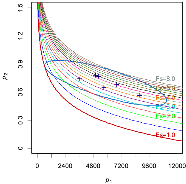
图 10 不同实际安全系数对应的极限状态线
