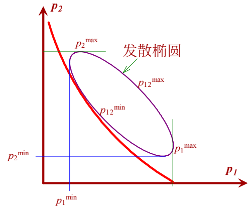
图 7 发散概率密度等值构型上的极限工况
