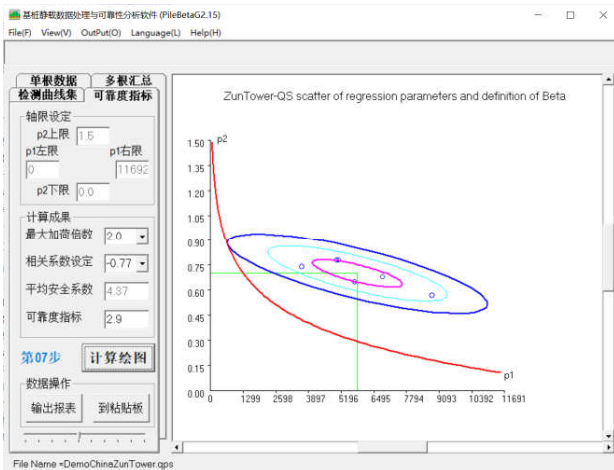
图9 回归参数的单倍标准差椭圆和发散椭圆
