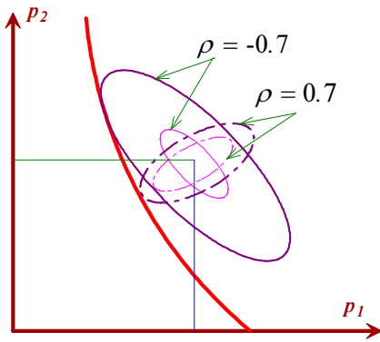
图 6 不同相关系数下概率密度等值构型的定义
