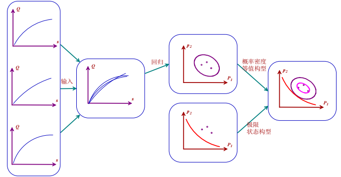
图4 基桩承载力几何可靠性分析流程
