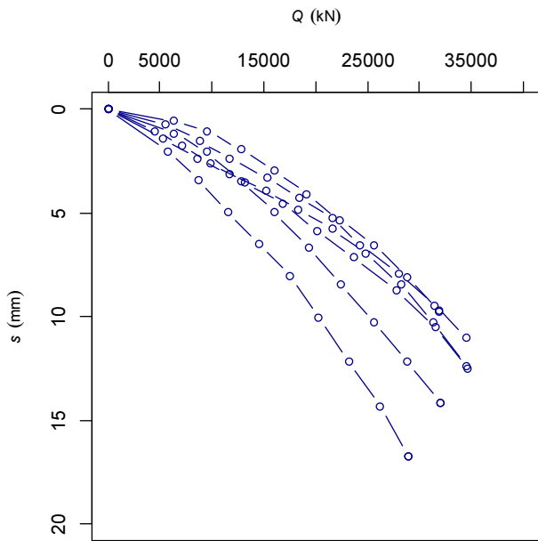
图8 中国尊大厦基桩的荷载-位移检测曲线
